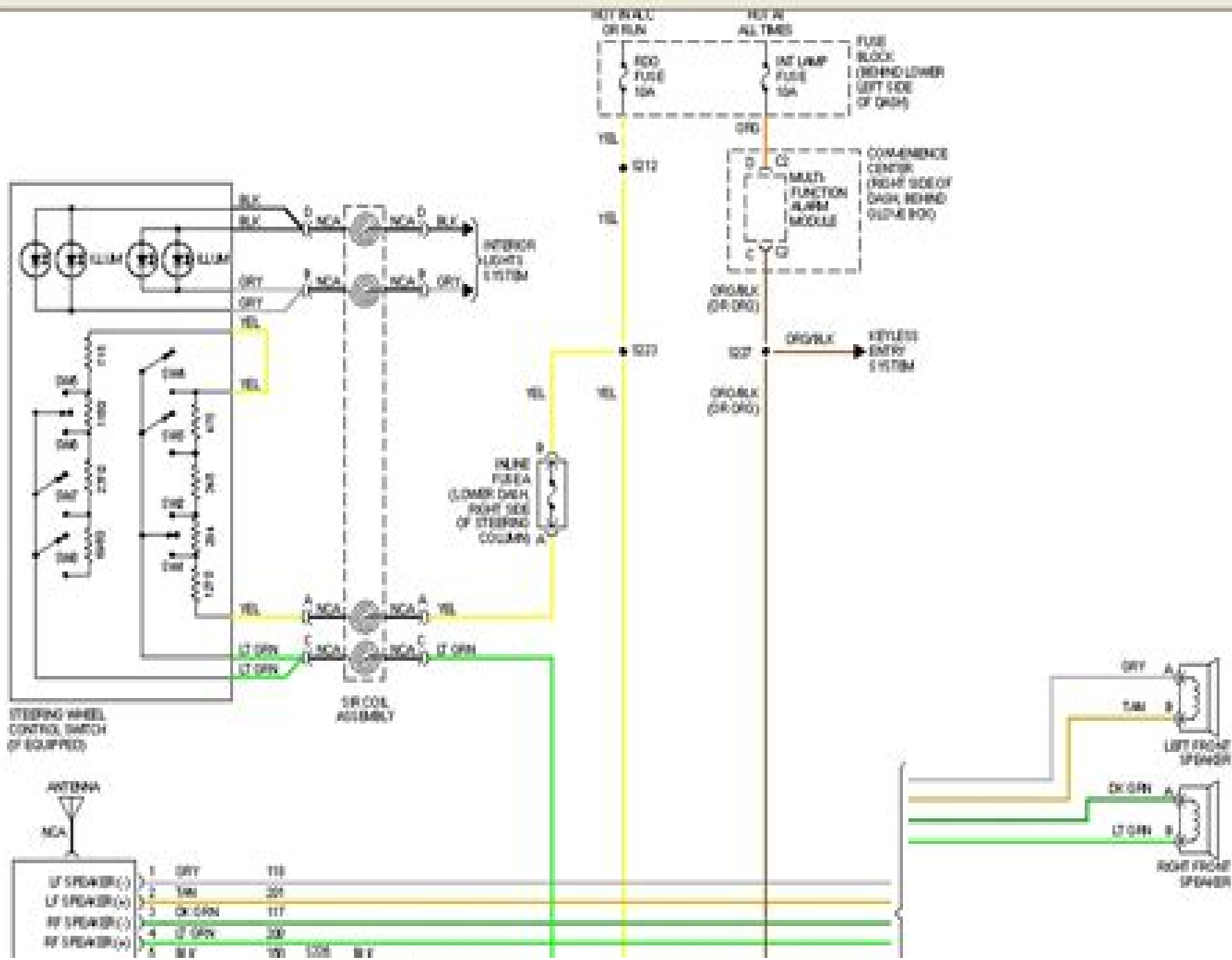
Fig. 34 Radio Circuits
