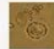
Entamoeba coli
