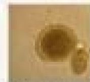
Tricostema caryi
