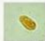
Giardia lamblia
