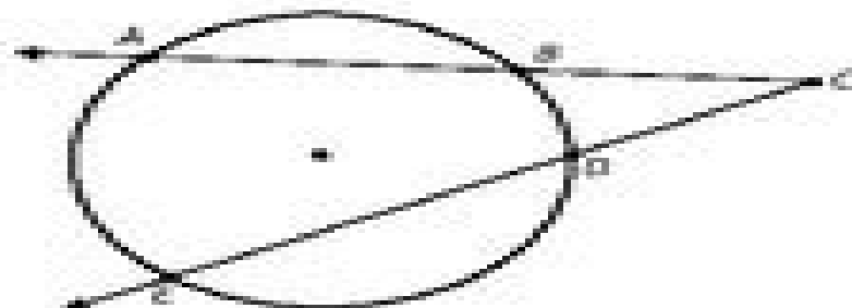
Secant-secant
