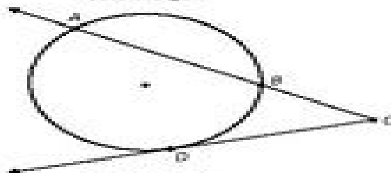
Secant-tangent
