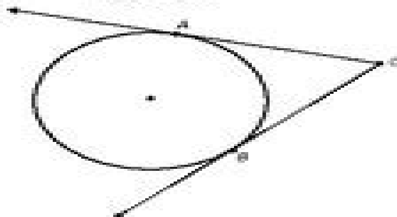
Tangent-tangent
