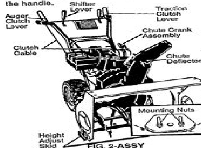
FIG. 2-ASSY
