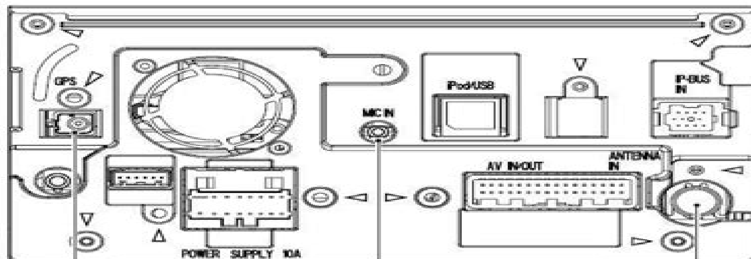
GPS ANTENNA
