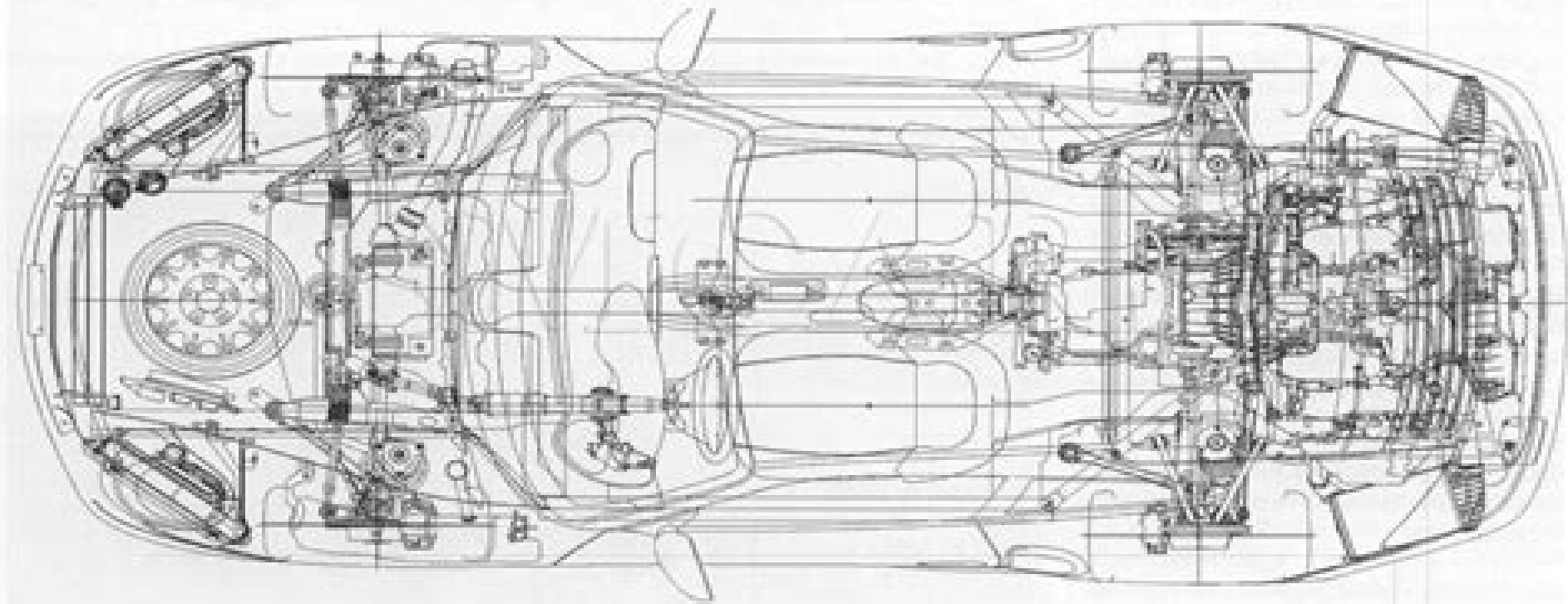
Bild 5: Package Draufsicht
