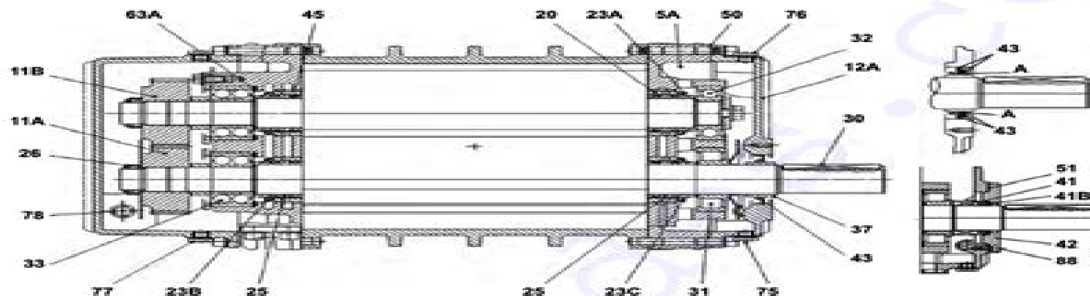
11.4 Sezione RBS 135-225
