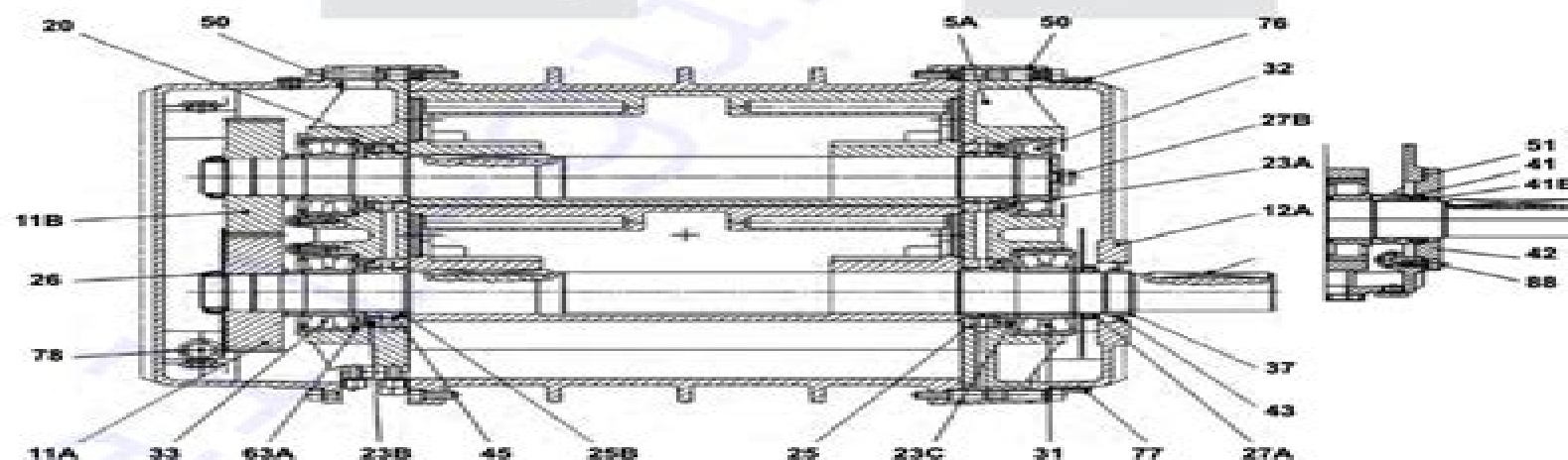
11.4 Sezione RBS 135-225
