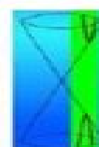
Hyperbola
